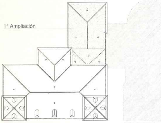
PLANTA DE CUBIERTAS ESTADO INICIAL
