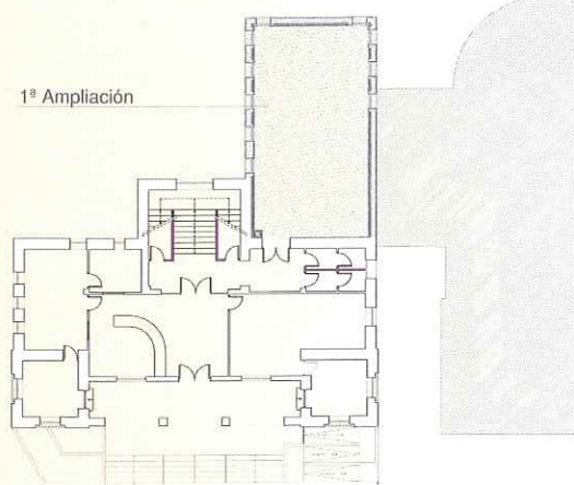
PLANTA BAJA ESTADO INICIAL
